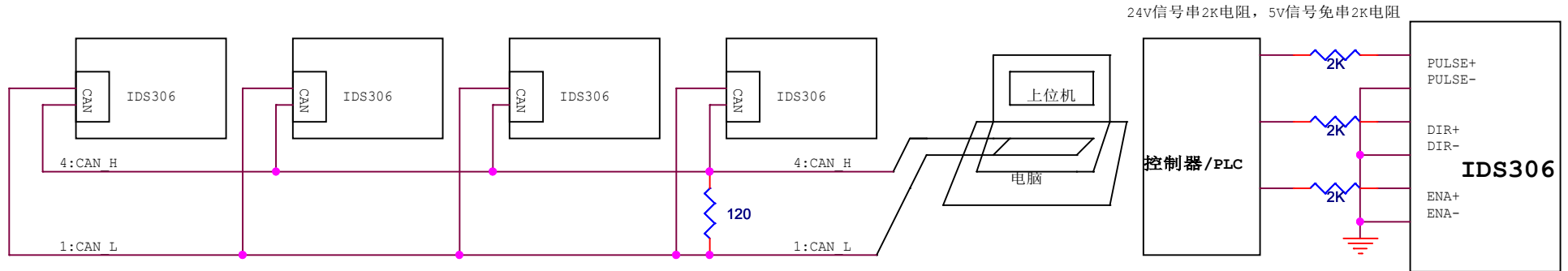
IDS306共阴极接法 (仅限于脉冲方向使能信号)
