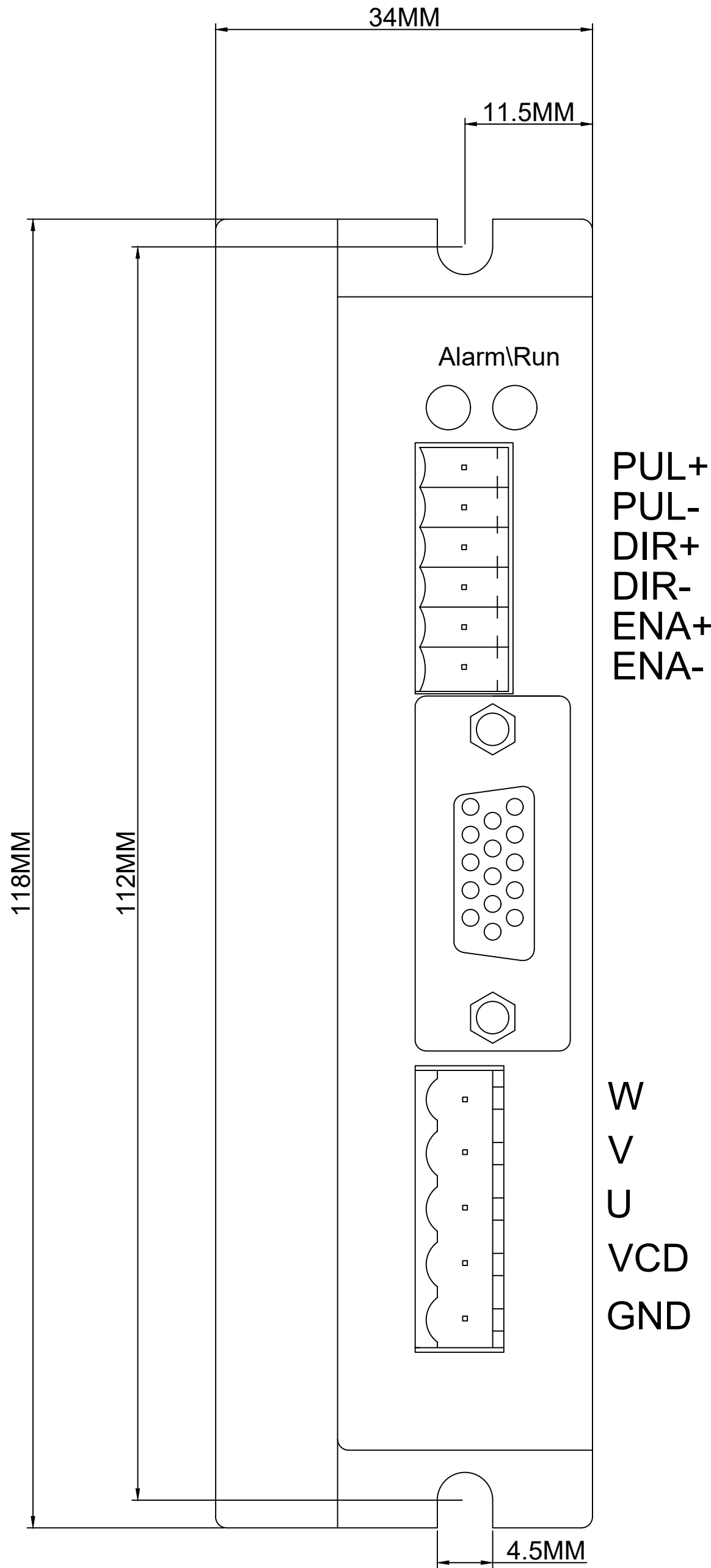
正面安装图
