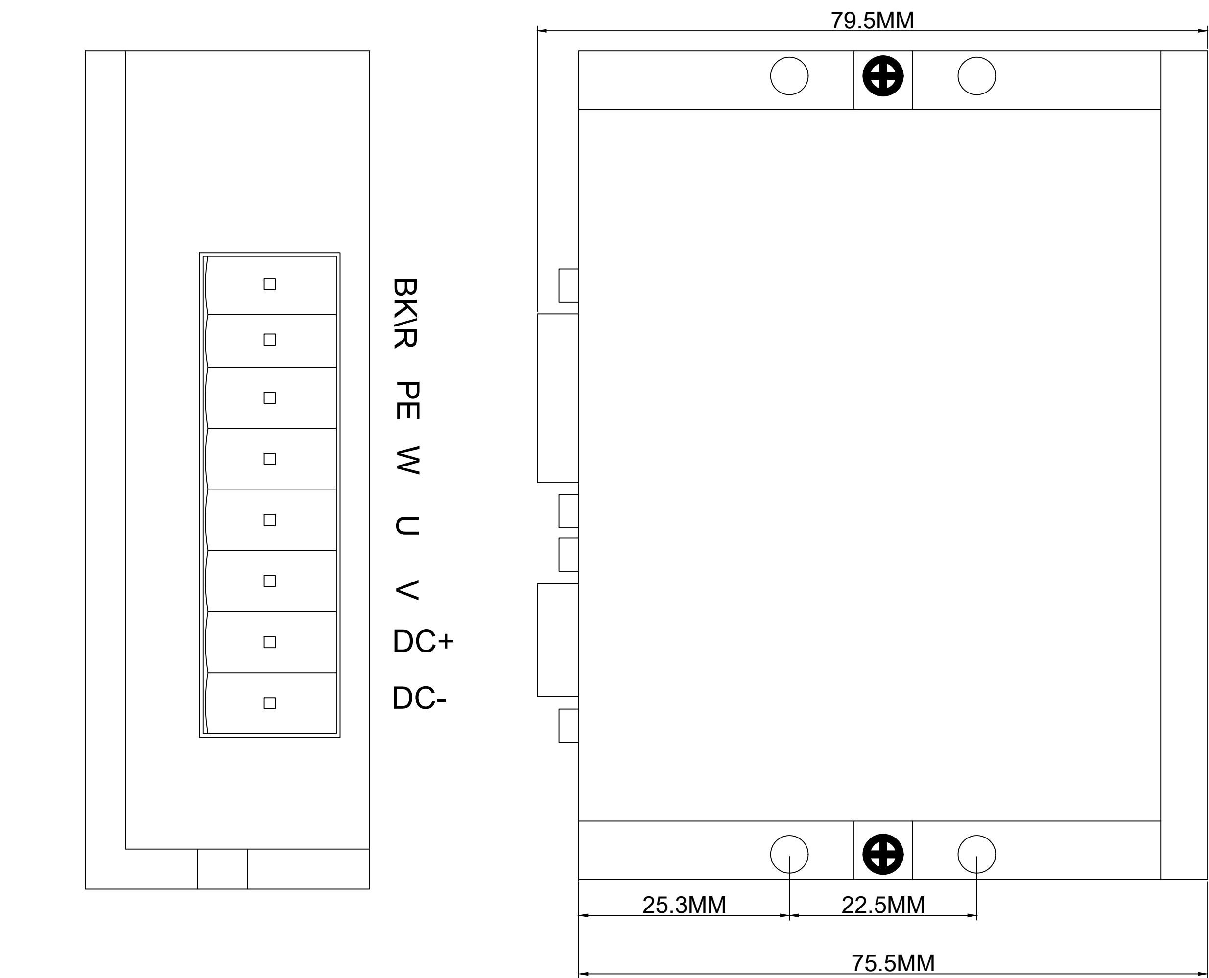
侧面安装图
