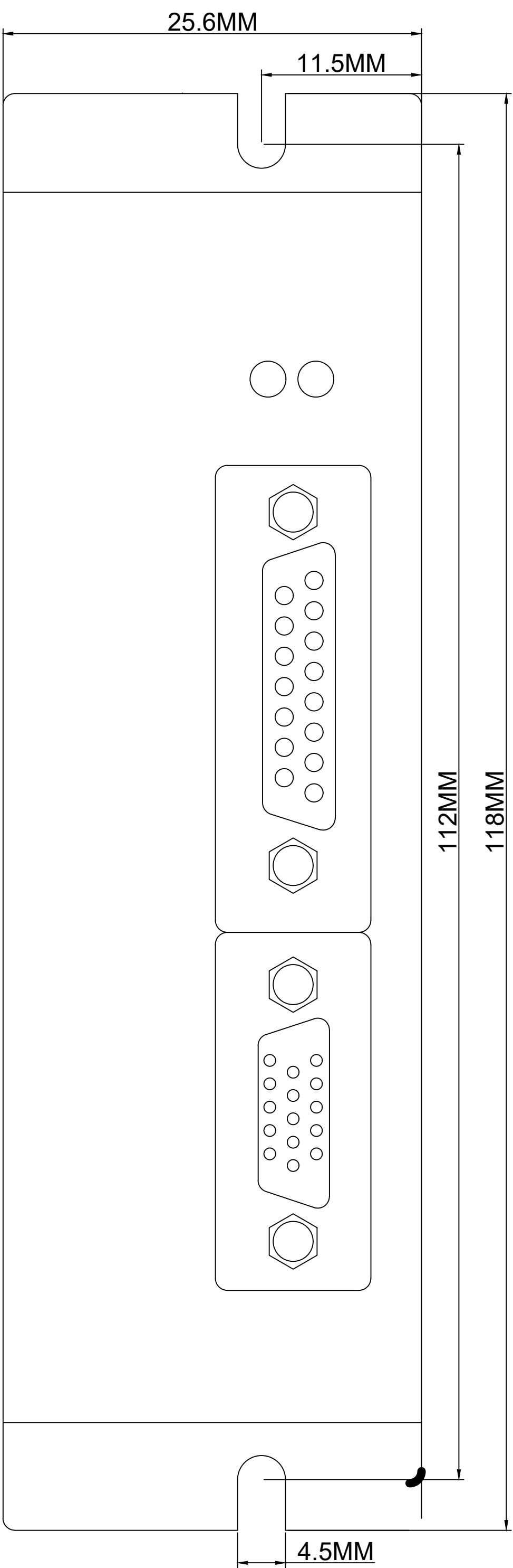
正面安装图
